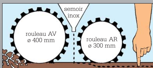
Le rouleau avant tasse et nivelle le sol
